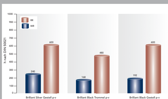
Korrosionsschutztafel
